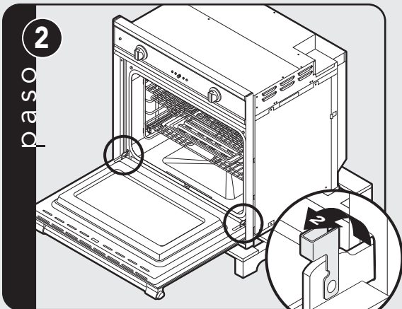
Abrir la puerta completamente. Gire la bisagra de la puerta a la posición desbloqueada.
