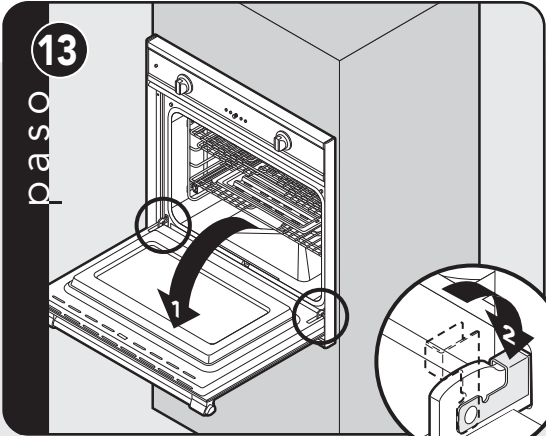
Abra la puerta completamente. Gire la bisagra de la puerta hasta la posición de bloqueo.
