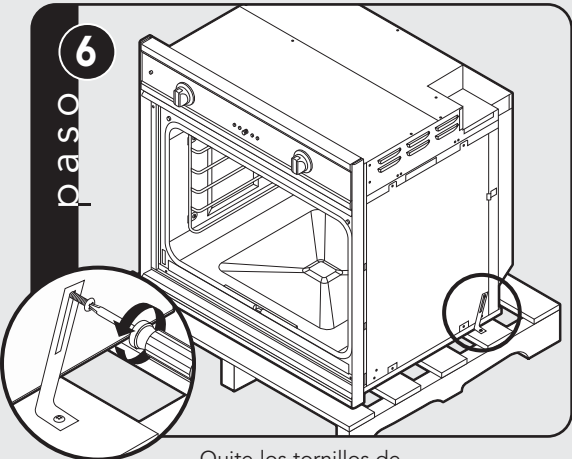
Quite los tornillos de la paleta desde la parte lateral del horno.
