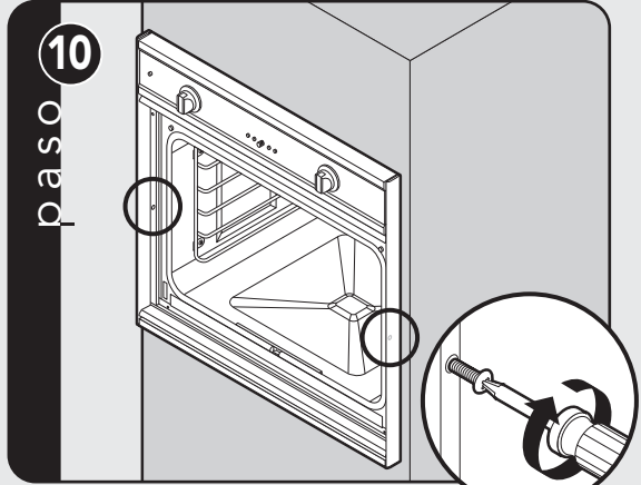
Instale los tornillos en el lado del bastidor. Nota: dos tornillos para los hornos sencillos y cuatro tornillos para los hornos dobles (no se incluyen los tornillos).
