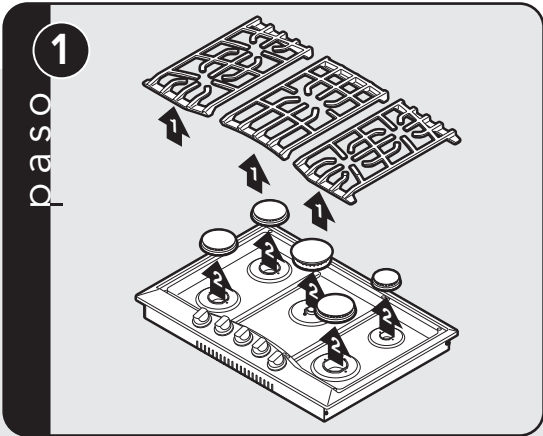
Retire las rejillas y las tapas de los quemadores.
