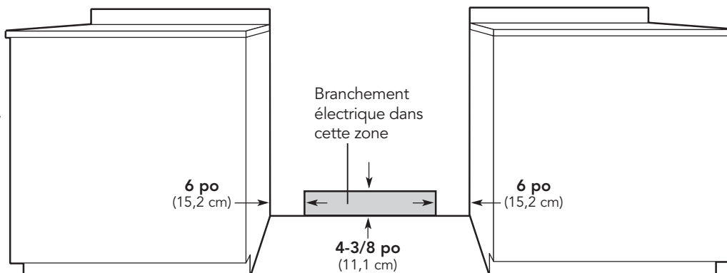
Cuisinière électrique 30"
