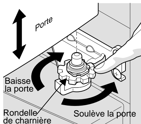
Monter ou abaisser la porte
