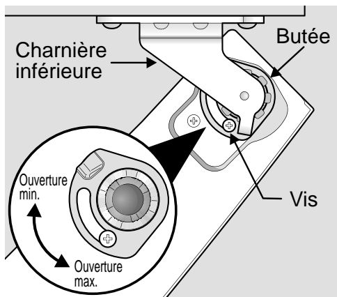
Butée de porte ajustable
