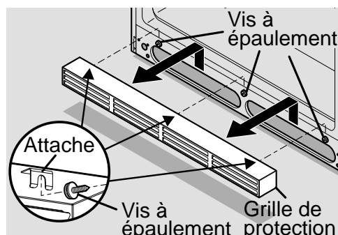
Figure 2 : Soulevez la grille de protection et tirez-la doucement vers l'avant.
