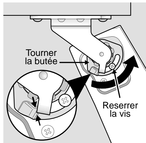
Resserrez la vis de pression
