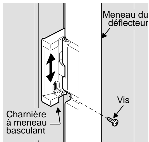
Réglage de la vis du meneau basculant
