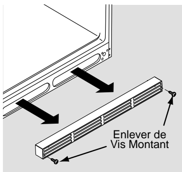
Figure 1 : Enlevez les vis et tirez doucement vers l'avant.
