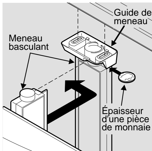
Réglage de la hauteur du meneau basculant
