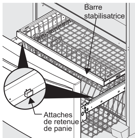
Les deux paniers du congélateur
