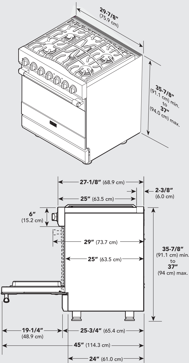
Cuisinière 30" W. à brûleurs mixtes
