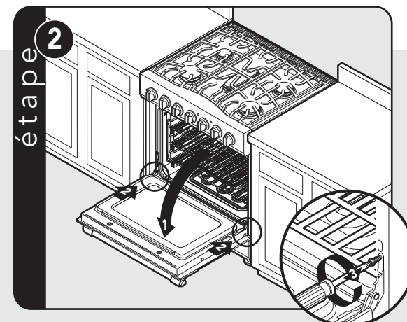
Ouvrez la porte complètement. Rattachez la garniture de charnière des deux côtés.
