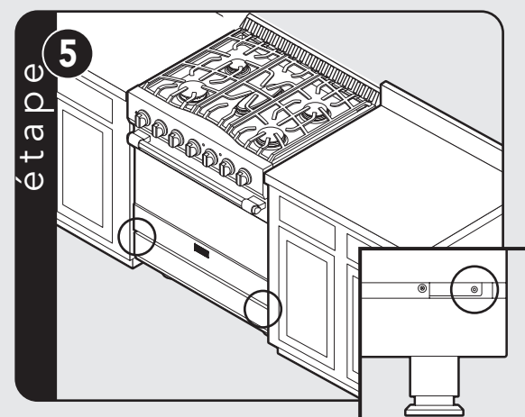
Si la porte doit être ajustée, desserrez les vis des garnitures de charnière situées à l'étape 2. Ajustez les vis qui se trouvent entre la porte et le garde-pieds à l'aide d'une clé Allen 5/32 po. Après l'ajustement, resserrez les vis des garnitures de charnière.
