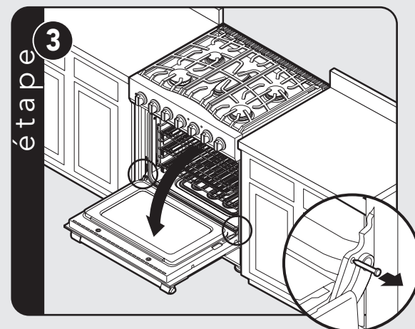
Retirez les goupilles des trous des charnières.
