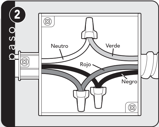
Conecte los cables rojo y negro del conducto de la unidad a los cables correspondientes en la caja de empalmes.
