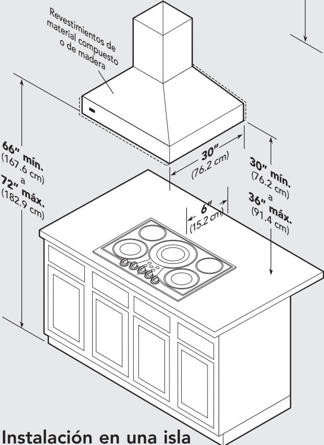
Instalación en una isla
