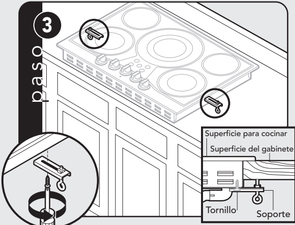
Atornille los soportes a la caja del quemador con un tornillo para metal. (Se incluyen dos conjuntos de soportes)
