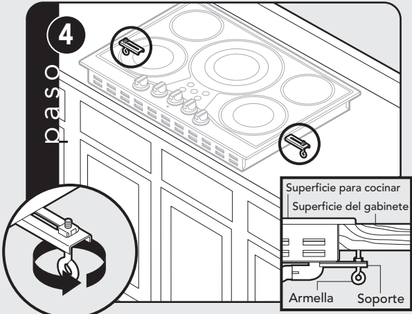
Atornille los tornillos en los soportes y apriételos firmemente contra la parte inferior de la superficie del gabinete. Nota: Tenga cuidado de no agrietar ni dañar el gabinete al apretar excesivamente los tornillos.
